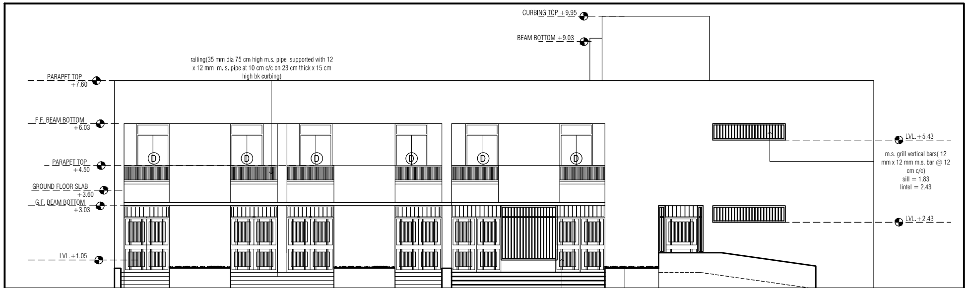
ELEVATION - A
