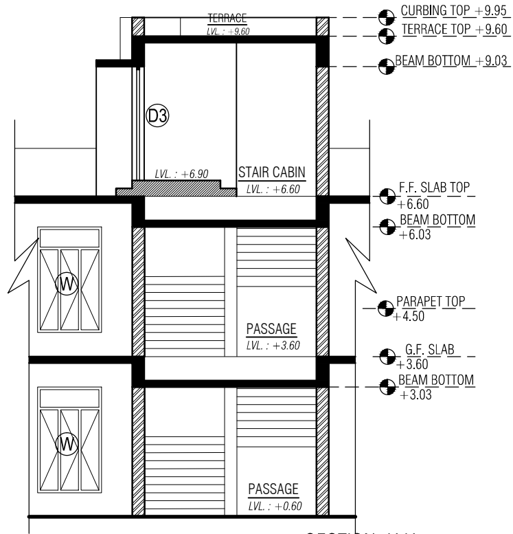
SECTION -X-X
